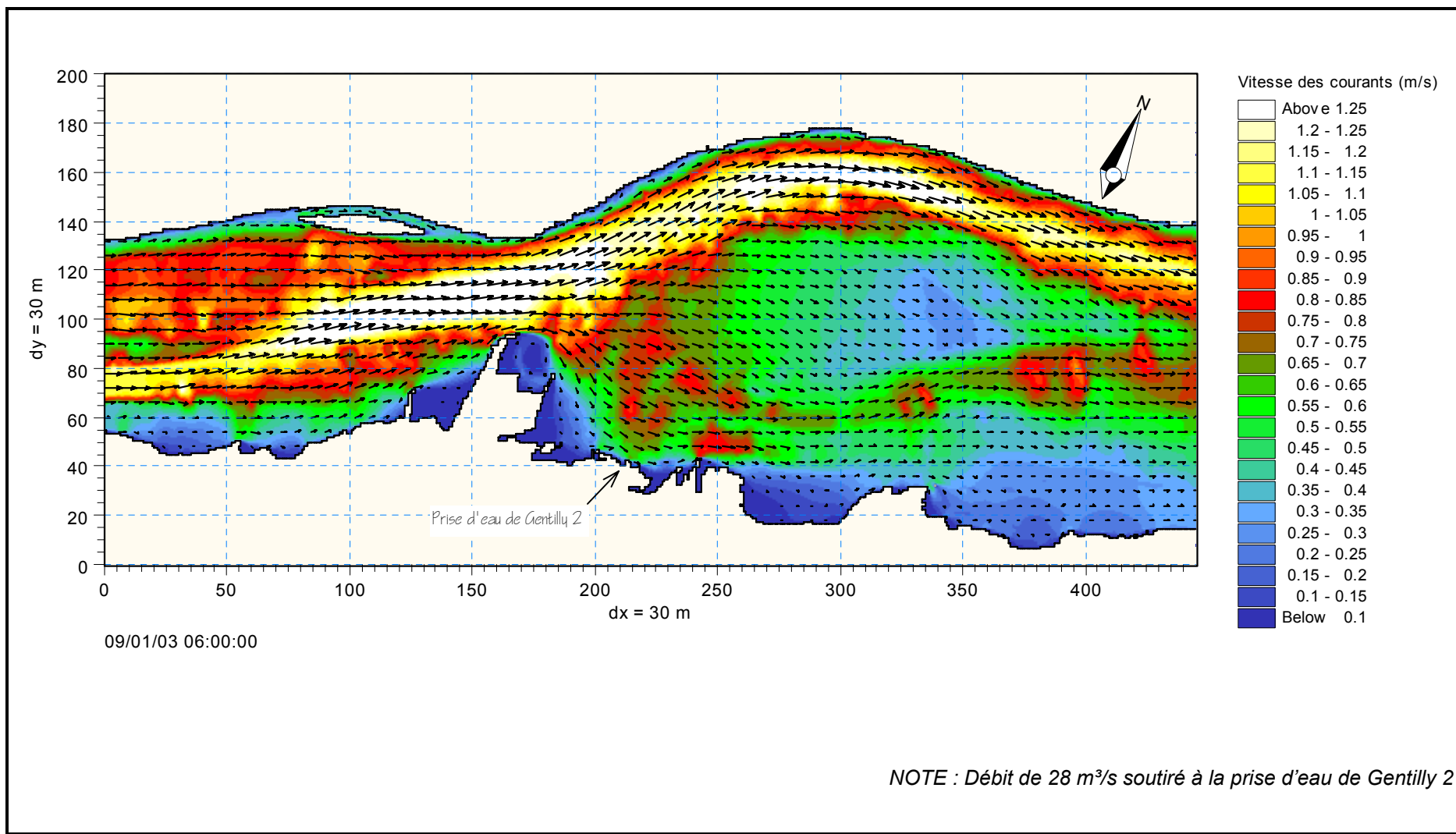
Figure 2.6 Champs de vitesse du fleuve – débit de crue
